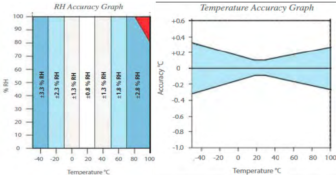
HMP155 产品特性曲线:
