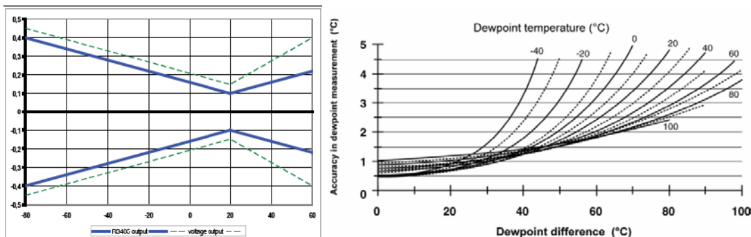
HMP155 产品特性曲线:
